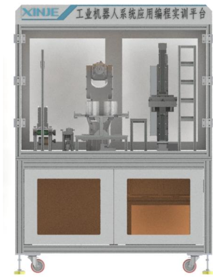
图 1 工业机器人系统应用编程实训平台
